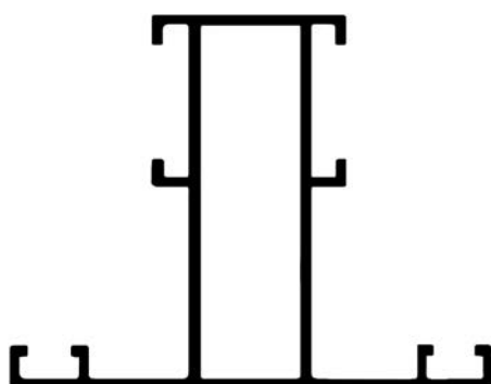
ALG M16 Travesaño paño fijo 0.700 kg/m
