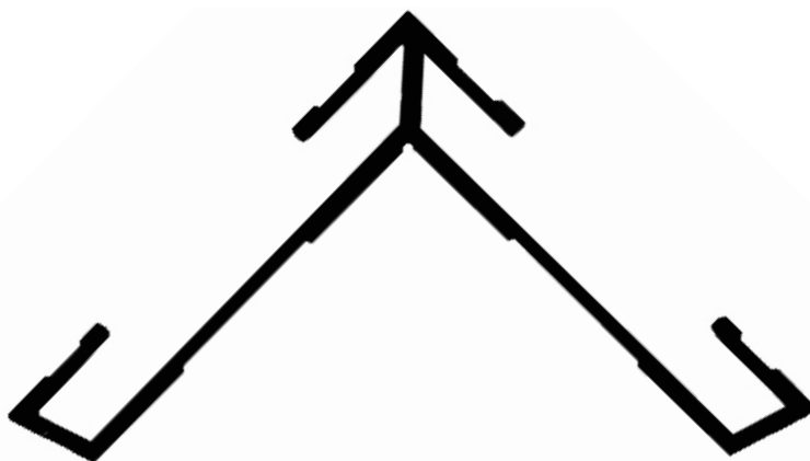
ALG 14.353 Escuadra de armado 1.558 kg/m
