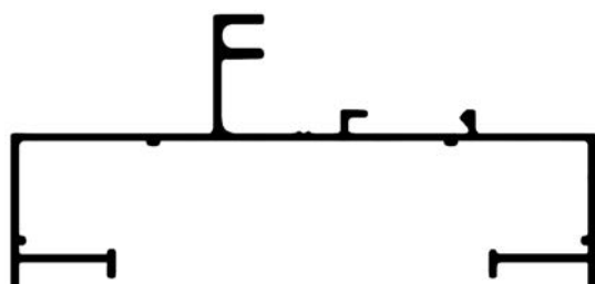
ALG N7 Marco paño fijo 0.580 kg/m
