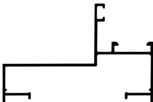
ALG 1176 Marco 75 mm 0.700 kg/m
