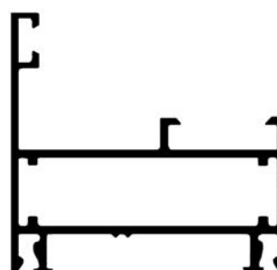
ALG M8 Marco ventana rebatir / paño fijo 0.720 kg/m
