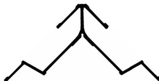
ALG 137 Escuadra de armado 0.595 kg/m
