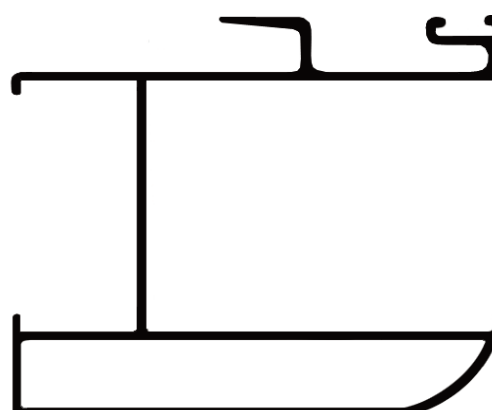
ALG 072 Parante central corrediza p/DVH 1.466 kg/m
