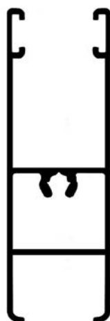
ALG R2 Zócalo / cabezal. Hoja corte a 90° 0.590 kg/m
