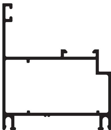
ALG 215 Hoja ventana borde recto / bandolera 0.864 kg/m
