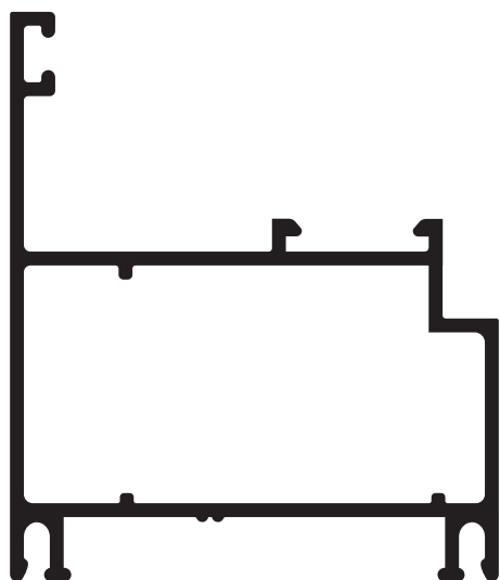
ALG 6040 Marco puerta de rebatir 1.180 kg/m
