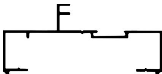
ALG N71 Marco paño fijo 0.620 kg/m
