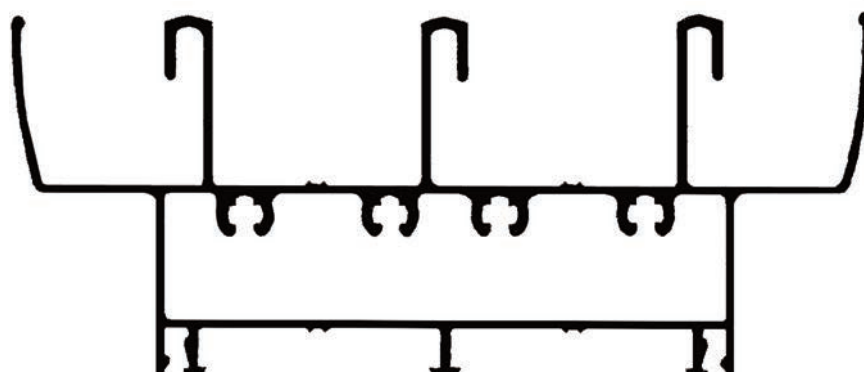
ALG M40 Umbral y marco de 3 guías 1.652 kg/m
