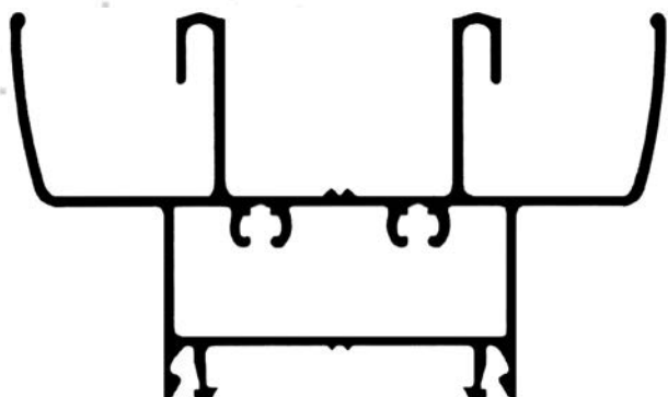
ALG M1 Umbral y dintel 1.250 kg/m
