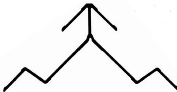
ALG 046 Escuadra de armado 0.690 kg/m
