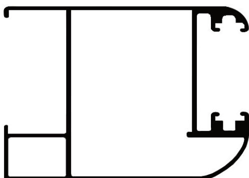
ALG 071 Parante lateral corrediza p/DVH 1.334 kg/m
