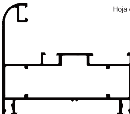
ALG 055 Marco paño fijo y ventana de abrir 1.037 kg/m
