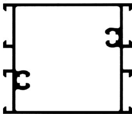
ALG M18 Travesaño puerta 1.01 kg/m
