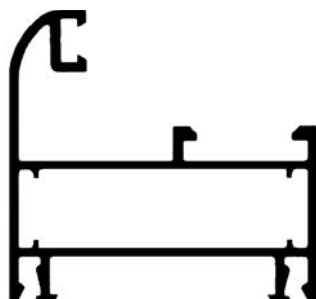
ALG M23 Marco / paño fijo curvo 0.760 kg/m
