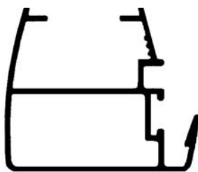
ALG 684 Corrediza Hoja Encuentro 0.380 kg/m
