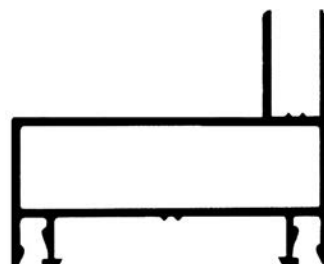
ALG M6 Jamba marco 0.610 kg/m
