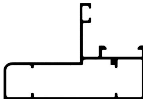
ALG 1160 Marco 64 mm 0.766 kg/m
