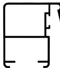
ALG R4 Parante central. Hoja corte a 90° 0.490 kg/m
