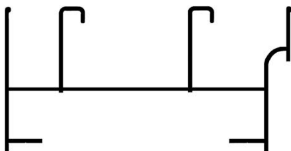
ALG N1/L Marco ventana corredizo 0.540 kg/m
