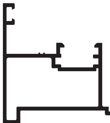
ALG 224 Encuentro central ventana de abrir 2 hojas 0.790 kg/m
