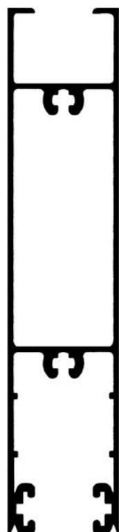
ALG M5 Zócalo alto vidrio simple 1.150 kg/m
