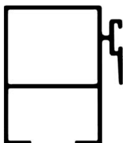
ALG M4 Parante central vidrio simple 0.580 kg/m
