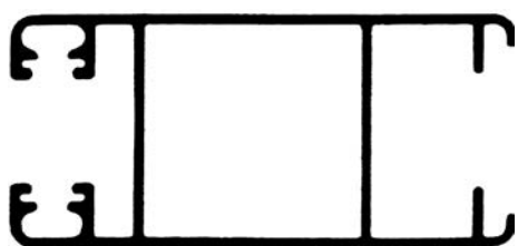
ALG R3 Parante lateral. Hoja corte a 90° 0.640 kg/m
