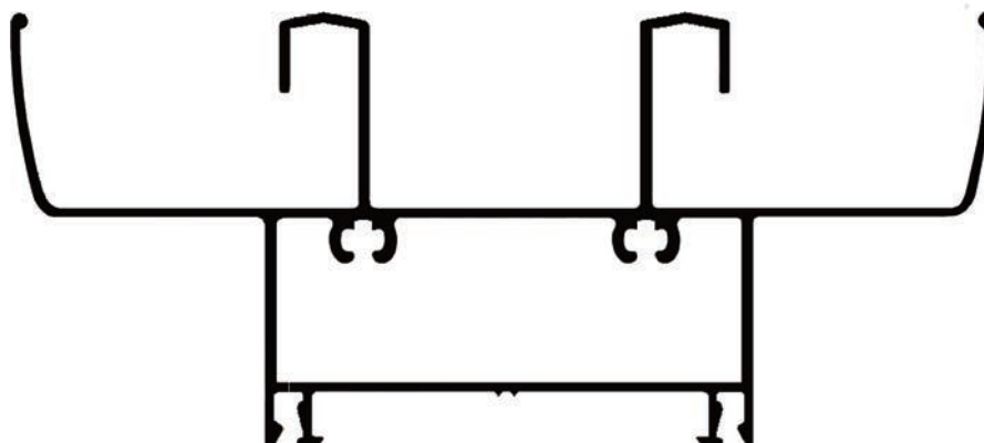
ALG 037 Umbral y dintel de marco 1.744 kg/m
