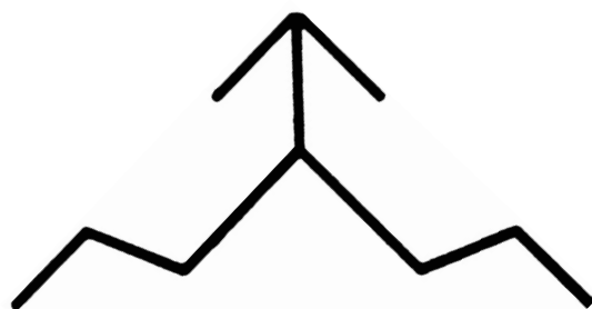
ALG 040 Escuadra de armado 0.398 kg/m
