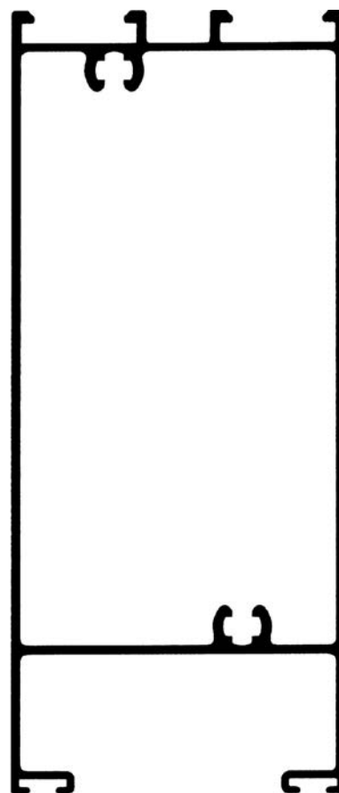
ALG M19 Zócalo puerta 1.610 kg/m
