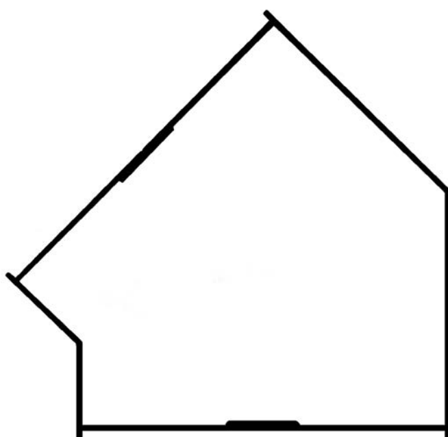
ALG 087 Acoplado 135° 1.304 kg/m
