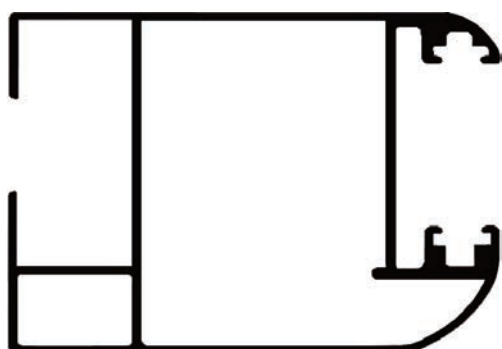
ALG 034 Parante lateral corrediza 1.399 kg/m
