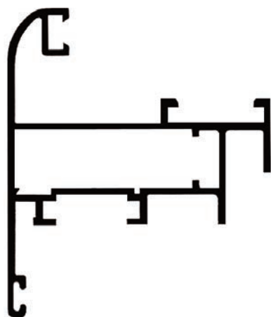
ALG M36 Hoja curva ventiluz 0.907 kg/m
