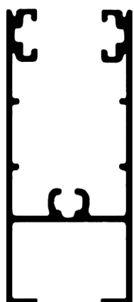
ALG M2 Zócalo y cabezal vidrio simple 0.680 kg/m
