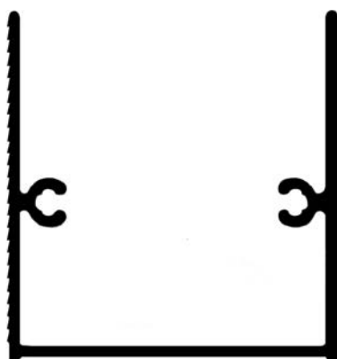
ALG 1405 "U" de armado 1.730 kg/m
