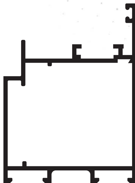
ALG 6041 Hoja puertas de rebatir 1.360 kg/m
