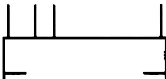
ALG 682 Corrediza Marco 90° Jamba 0.581 kg/m
