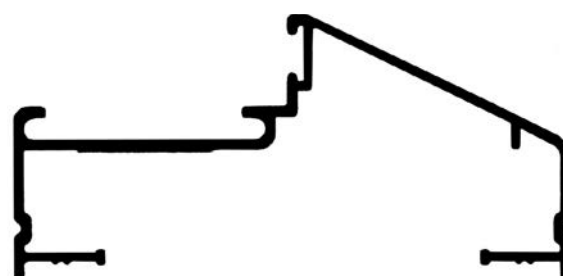
ALG 199 Marco puerta 36mm 0.580 kg/m
