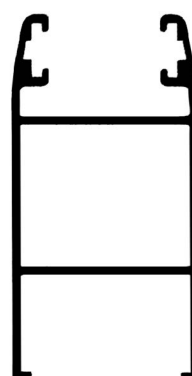
ALG M13 Parante lateral DVH 0.630 kg/m
