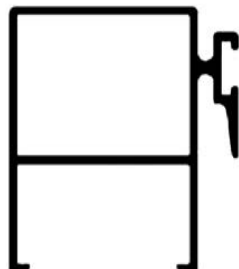
ALG M14 Parante central DVH 0.580 kg/m
