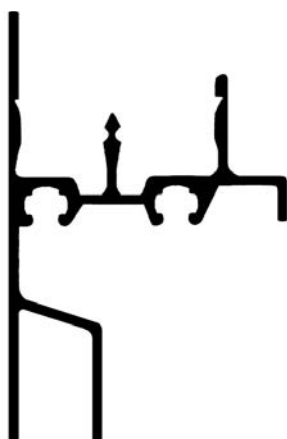
ALG 2002 Travesaño ventanilla 0.840 kg/m
