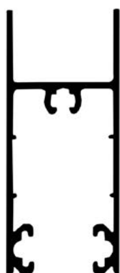
ALG M12 Zócalo y cabezal DVH 0.670 kg/m
