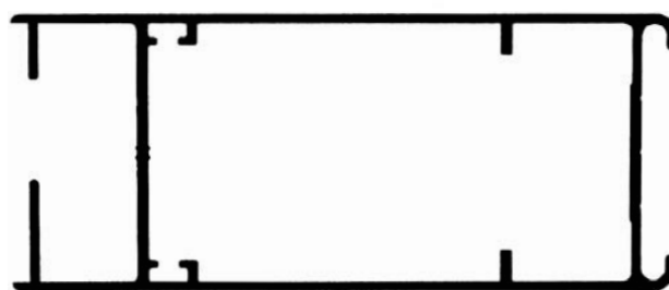
ALG 200 Parante puerta 36mm 0.986 kg/m
