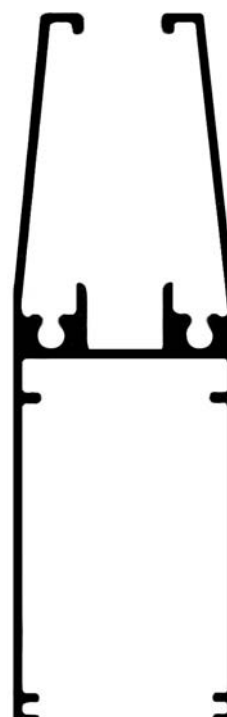
ALG 089 Zócalo para vidriado 1.790 kg/m
