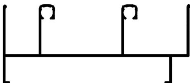
ALG 681 Corrediza Marco 90° Umbral/Dinte 0.691 kg/m
