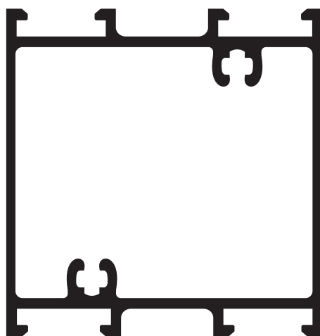
ALG 6042 Travesaño puerta de rebatir 1.380 kg/m
